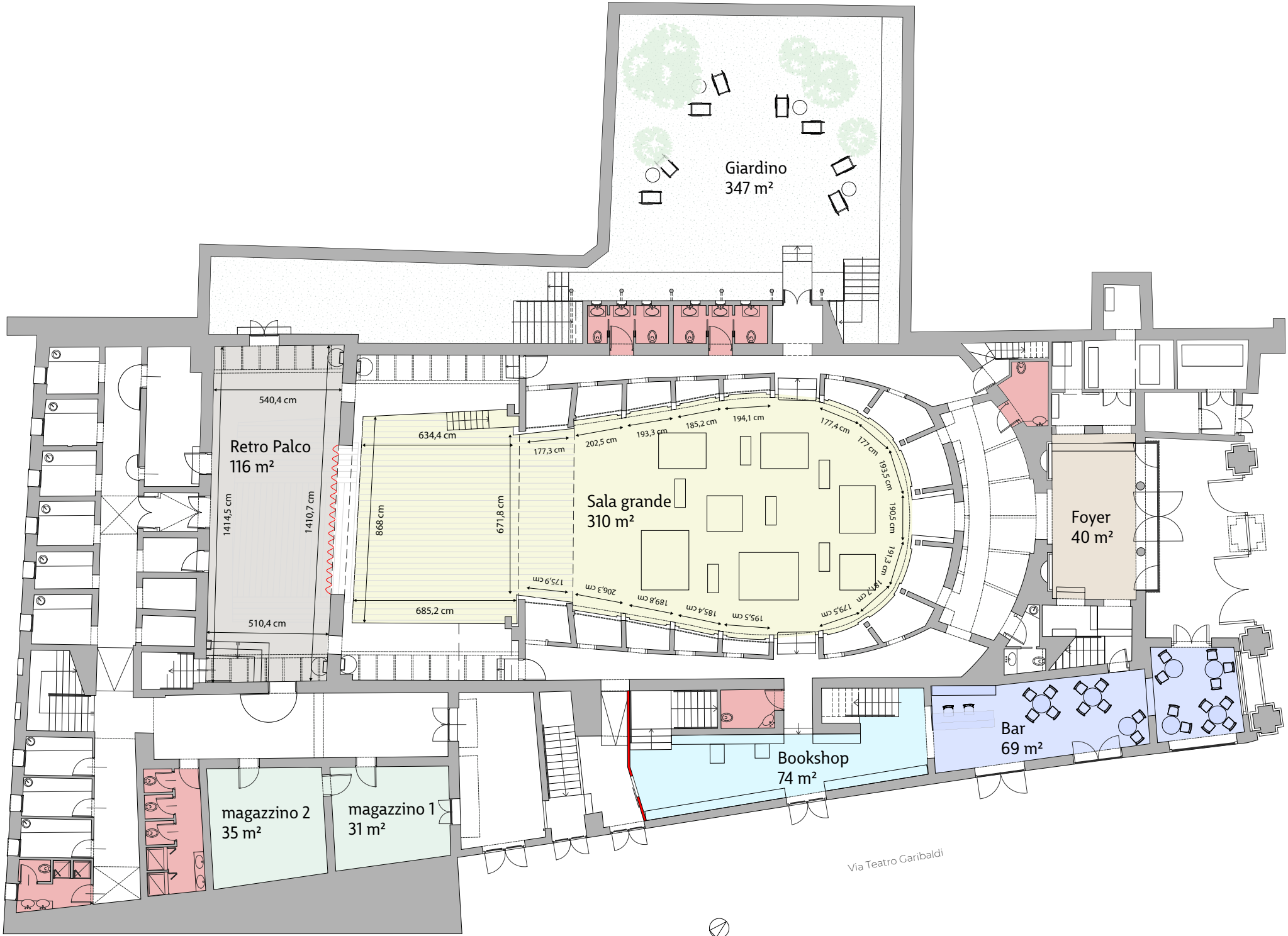
Teatro Garibaldi Legenda spazi Pianta a + 1.50 Scala 1:200
